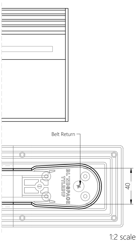
RETURN BOX TTSRB1F & HEAD BOX
