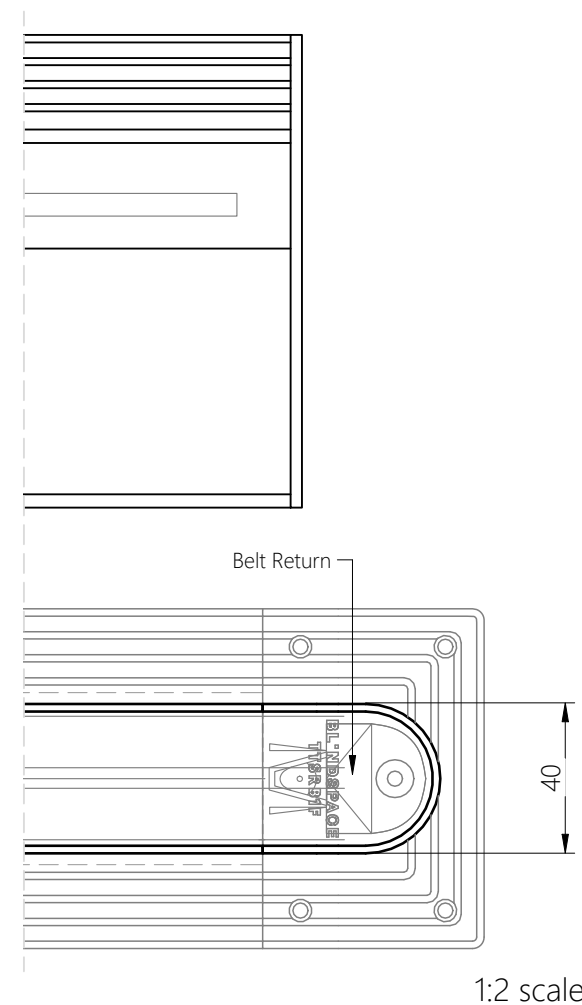
RETURN BOX TTSRB1F & HEAD BOX
